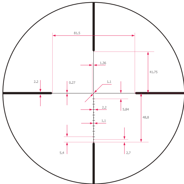
2.5-20X56 PRO Reticle
