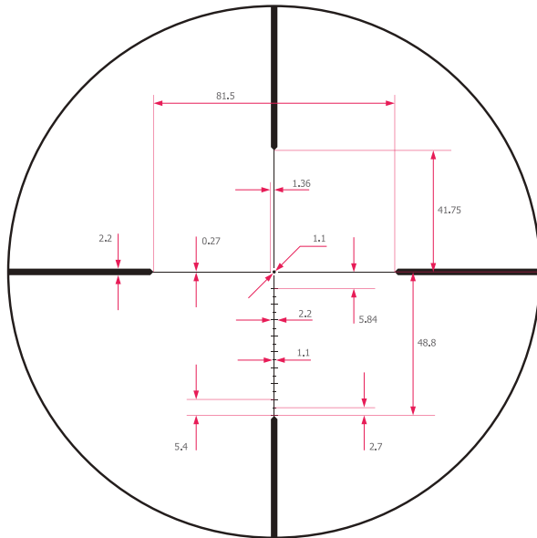
2.5-20X50 PRO Reticle
